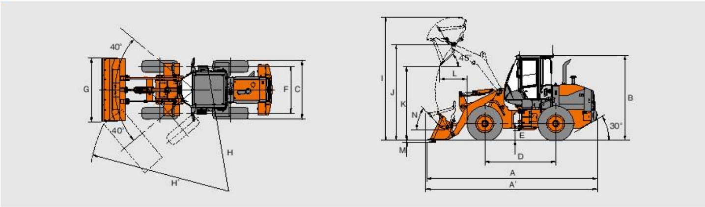
■ 寸法図
